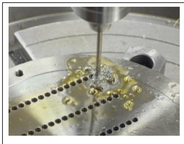
加工の様子（リーマによる穴仕上げ）
